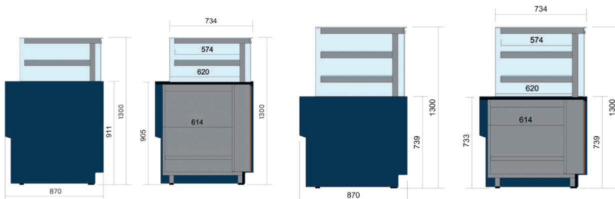
Versions 2 niveaux / soubassement haut
