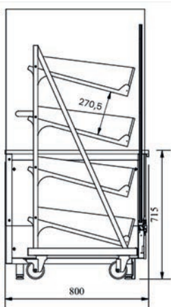
Encombrement total
