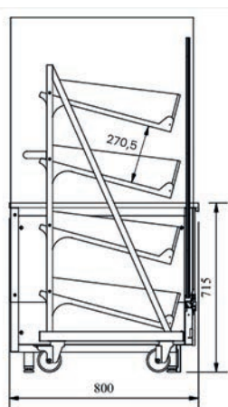
Encombrement total
