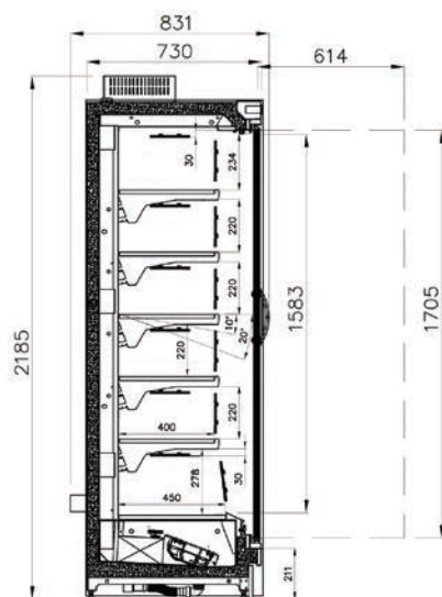
Vitrine avec groupe logé 2 portes
