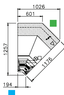
ANGLE 45° : INTÉRIEUR
