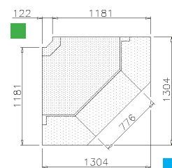
ANGLE 90° : EXTÉRIEUR
