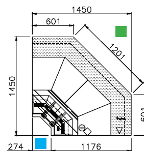
ANGLE 90° : INTÉRIEUR
