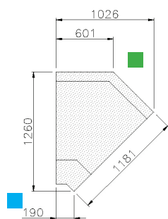
ANGLE 45° : INTÉRIEUR
