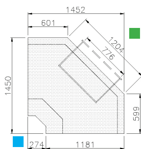
ANGLE 90° : INTÉRIEUR
