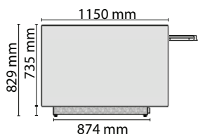
Meuble caisse PMR
