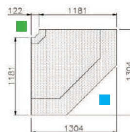
ANGLE 90° : EXTÉRIEUR
