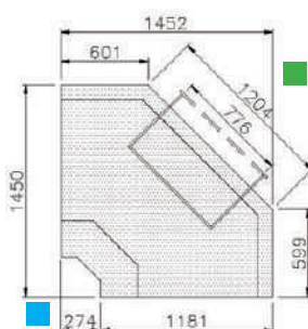
ANGLE 90° : INTÉRIEUR
